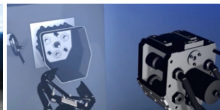
Połączenie CEJN do zdalnie kierowanych pojazdów podwodnych do zastosowań offshore.
