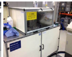
Stanowiska do badania ciśnienia impulsowego do 4000 bar.
